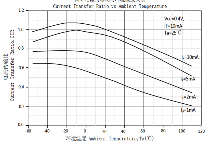
图8. 电流传输比与环境温度关系
