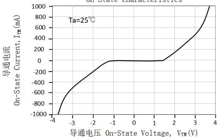
图2. 导通特性 On-State Characteristics
